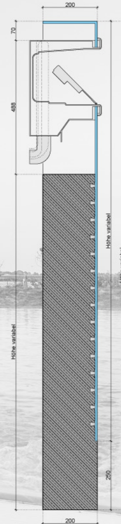
Systemschnitt 2.11 Wandelement mit Skimmer
