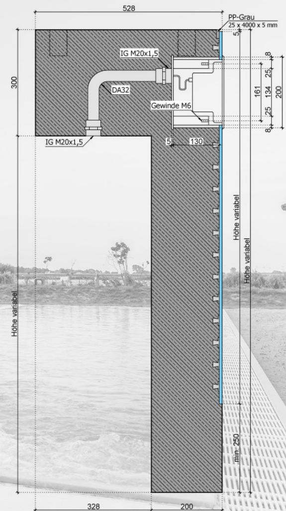
Systemschnitt 2.3 Wandelement mit UWS Anschluss nach unten
