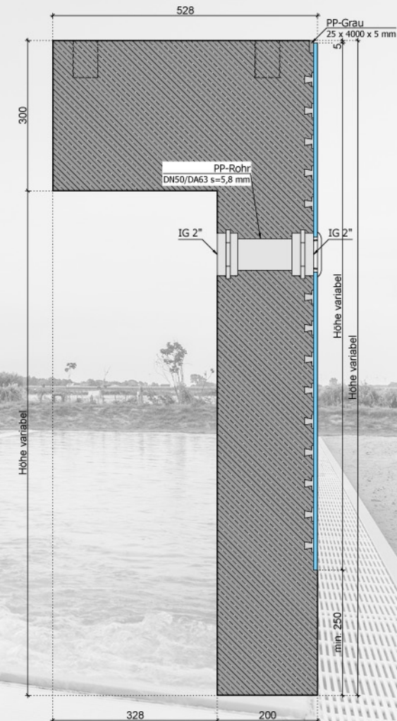
Systemschnitt 2.5 Wandelement mit Einströmdüse Anschluss über IG
