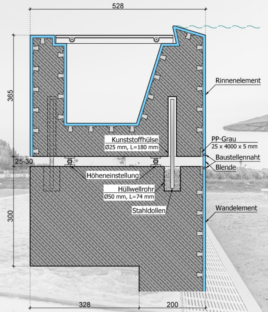
Systemschnitt 3.2 Anschluss Rinnenelement zum Wandelement
